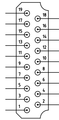
HDMI
