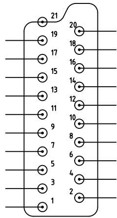
scart
