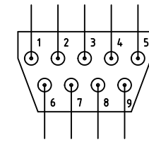
RS-232 socket
