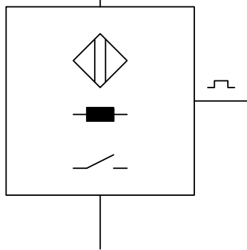
NO kapazitiv
