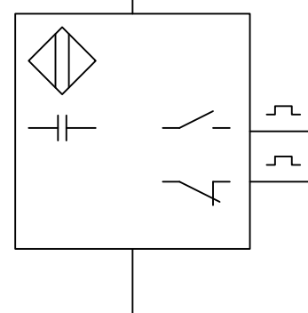
NO/NC Lichtschranke
