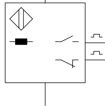
NO/NC kapazitiv
