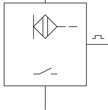
NO ultraschall
