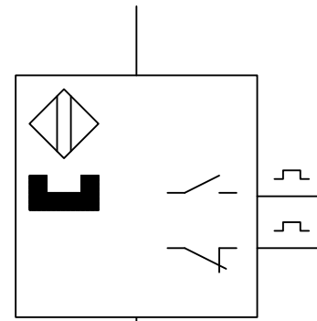
NO/NC Zylinderschalter
