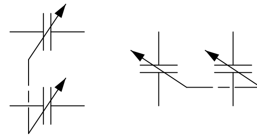
Drehkondensator, mehrfach
