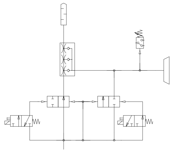
Vakuum Ejektor
