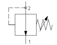
Vakuumregelventil vertikal
