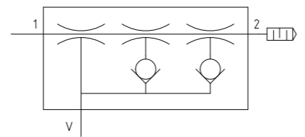
Vakuum Ejektor mehrstufig
