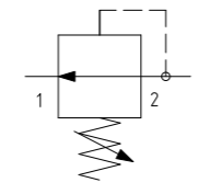
Vakuumregelventil horizontal
