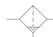
Filter, autom. Kondensatablass
