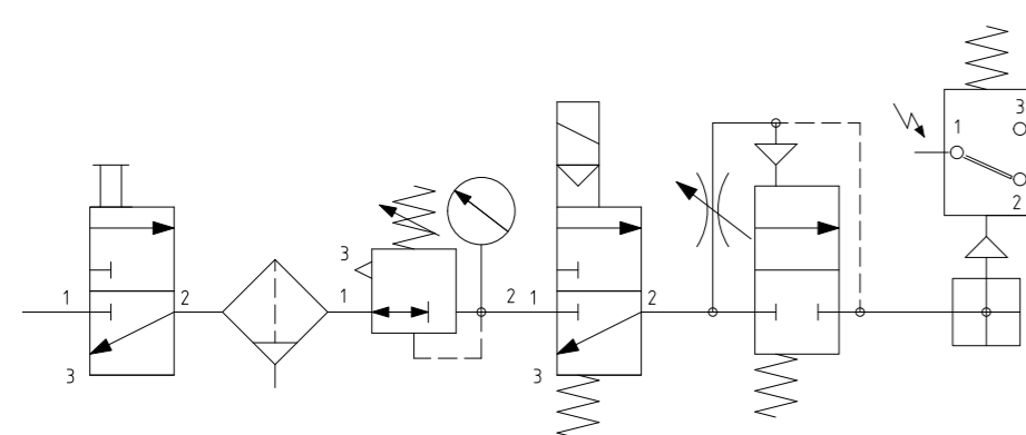
Wartungseinheit, mit Absperrventil, elektr. Einschaltventil, Softstart, Druckschalter
