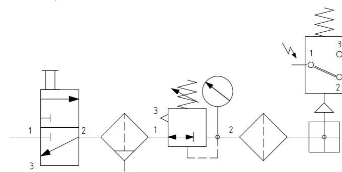
Wartungseinheit, mit Absperrventil, Feinfilter, Druckschalter
