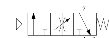
Softstartventil 3/3 WV - pneumatisch - horizontal
