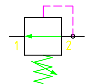
Vakuuregelventil horizontal
