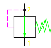
Vakuuregelventil vertikal
