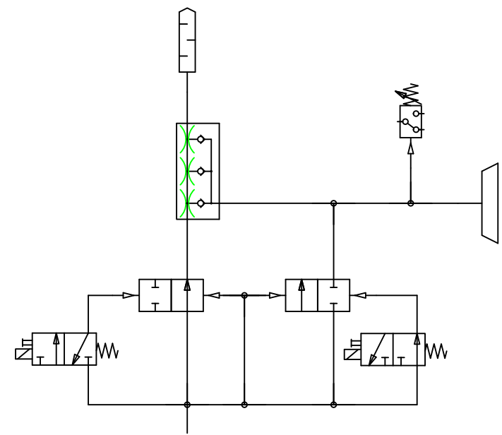
Vakuu Ejektor
