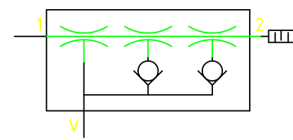
Vakuu Ejektor mehrstufig
